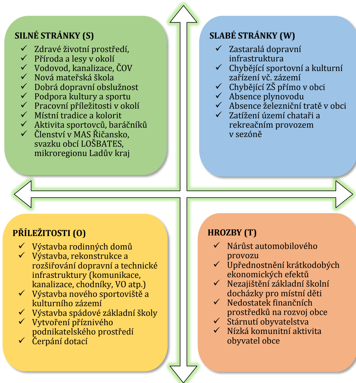
Obrázek 18: Matice SWOT
